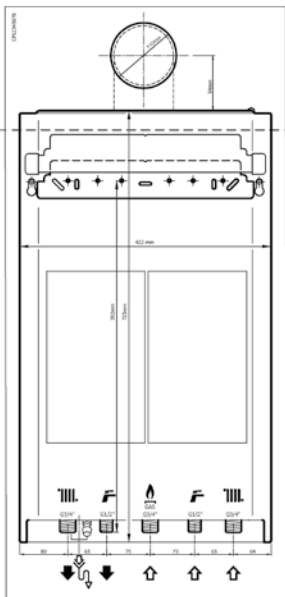
Рисунок 1. Шаблон/схема монтажа
