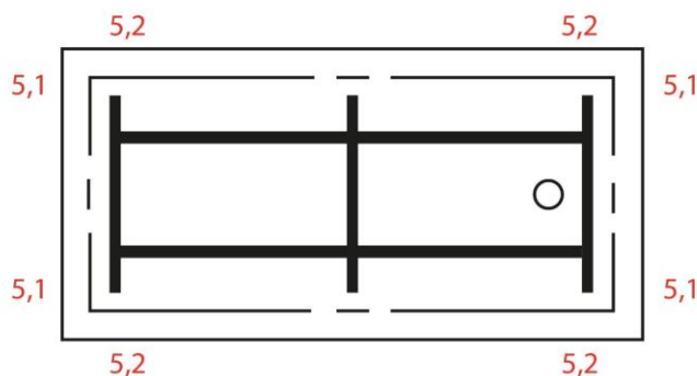
уголок (металл)
